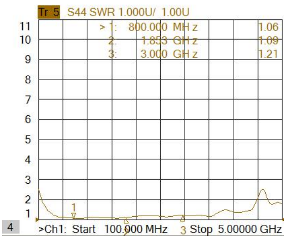
图 4 输出端驻波测试结果
