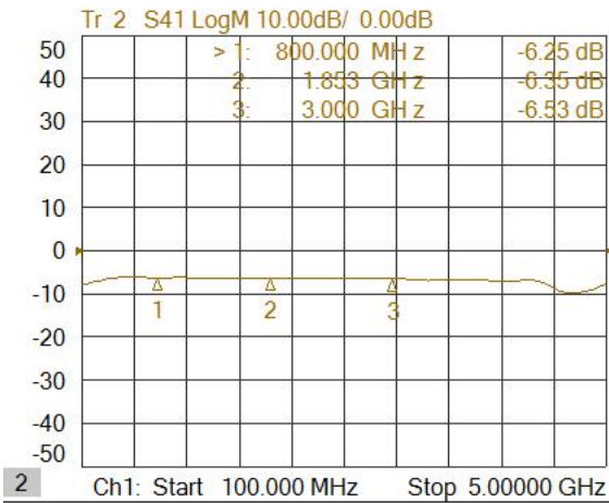
图 1 插入损耗测试结果
