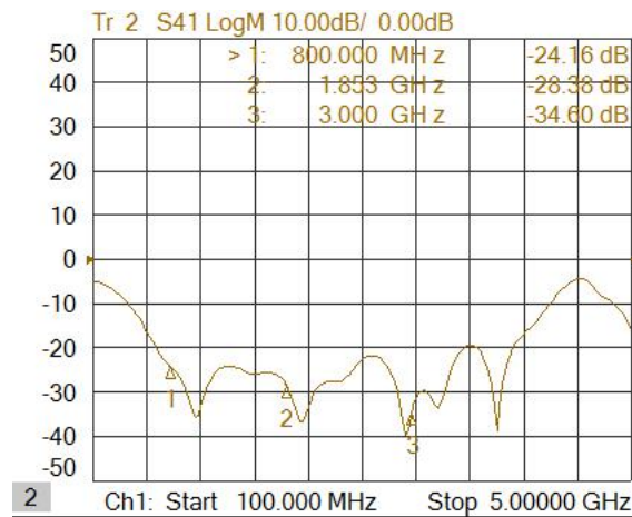
图 3 隔离度测试结果
