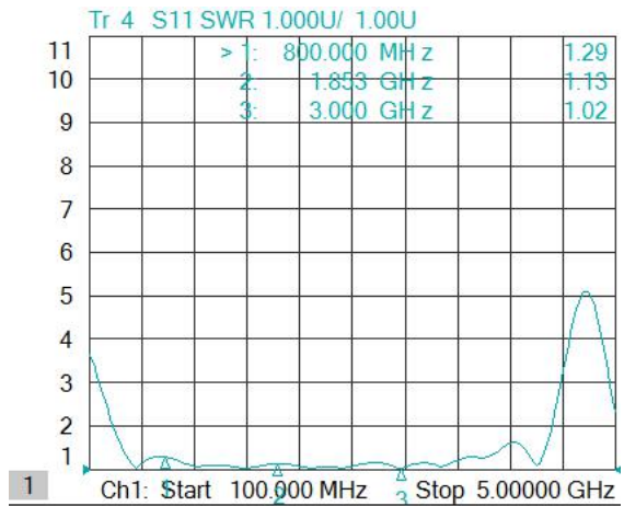
图 2 输入端驻波测试结果
